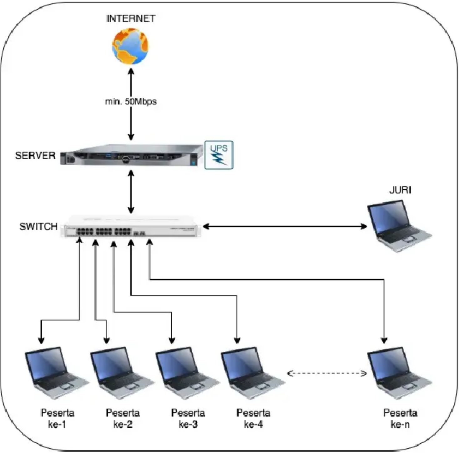
Gambar 1. Topologi jaringan untuk lomba.
